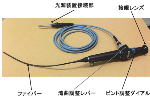
図1 内視鏡の構造
