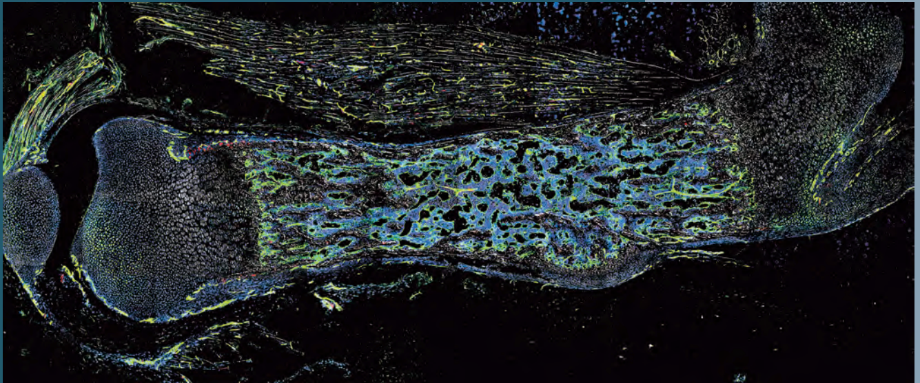
マウス大腿骨(3日齢)の凍結切片を共焦点レーザー顕微鏡で観察した画像。青色は核、緑は血管(CD31陽性血管内皮細胞)を染色している。骨髓の血管は、骨代謝の調節において重要な役割を担う。
